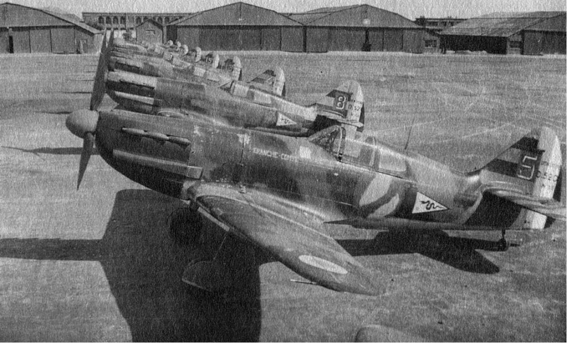
La Sénia, 1941 – Dewoitine 520 du GC I/3 – Les marques distinctives de l'aviation d'Armistice sont visibles sur les empennages (Raymond Macia)
